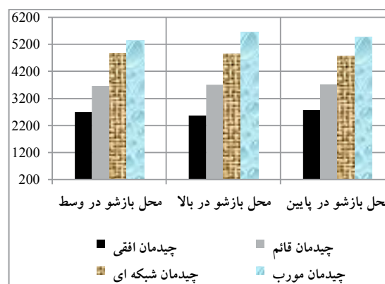
شکل ۳۱ مقایسه تاثیر چیدمان آرماتور روی مقاومت نهایی تیرهای با ابعاد بزرگ
