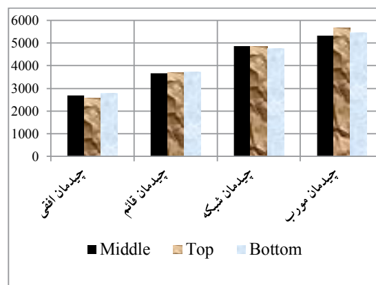
شکل ۳۰ تاثیر محل بازشو روی مقاومت تیرهای با ابعاد بزرگ
