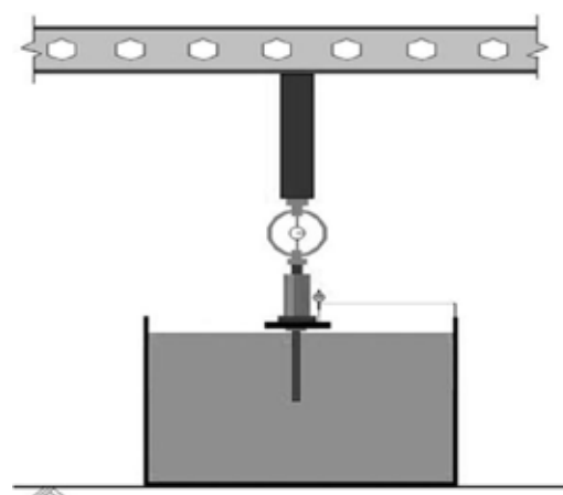
شکل ۳: دستگاه ظرفیت باربری
