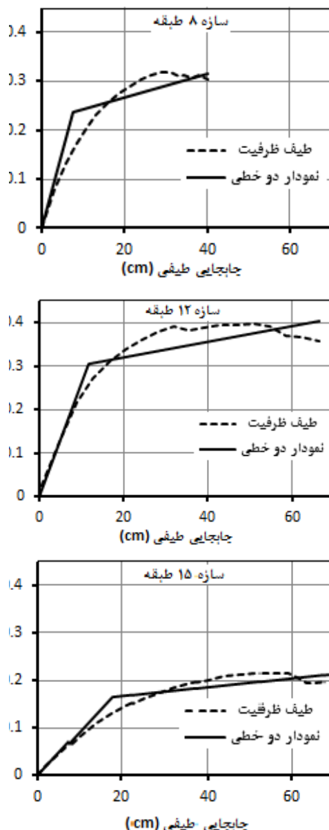
شکل ۱- منحنی ظرفیت و نمودار دوطبقی سازه‌ها
