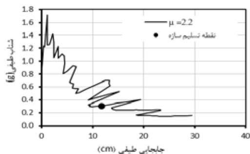
شکل ۸- نحوه تعیین پاسخ در روش YPS
