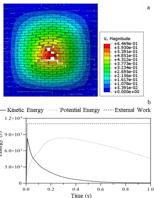
شکل ۴. الف) کانتور تغییر شکل و ب) نمودار انرژی دیوار
