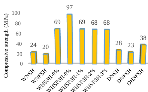
شکل ۶. مقاومت فشاری ۲۸ روزه طرح اختلاط‌های بتن پاششی
