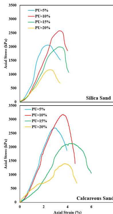
شکل ۵. نتایج آزمایش‌های تک محوری بر روی نمونه‌های تثبیت شده با پلی‌ارتان
