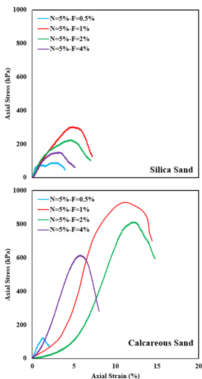
شکل ۴. نتایج آزمایش‌های تک محوری بر روی نمونه‌های تثبیت شده با
