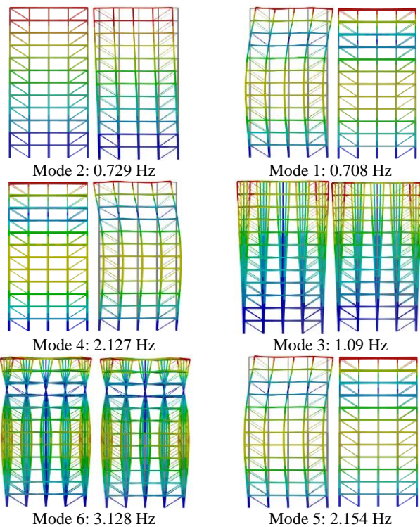
شکل ۹. فرکانس طبیعی ساختمان ۱۲ طبقه در حالت استفاده از میراگر از نمای روبرو و جانب.
