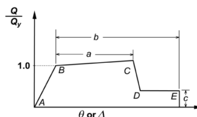
شکل ۴: منحنی نیرو-تغییر شکل تعمیم یافته برای اعضا و اجزای فولادی
