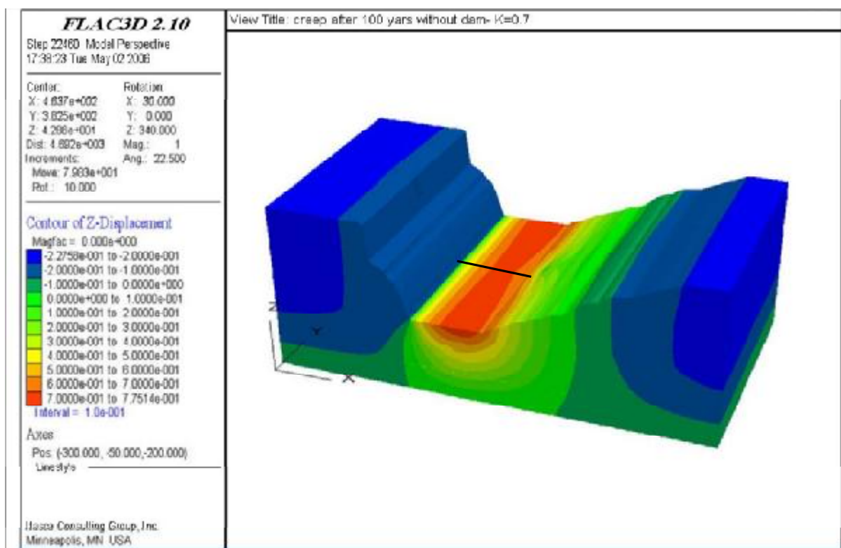
شکل (۷) خطوط تراز جابجایی‌های قائم پس از خزش ۱۰۰ ساله بدون اعمال وزن سد برحسب متر برای K=0/7
