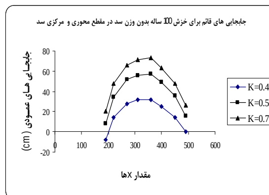
شکل 8 مقادیر جابجایی‌های عمودی برای چند نقطه روی سطح پی در مقطع محوری و مرکزی برای مقادیر مختلف K برای خزش 100 ساله بدون اعمال وزن سد
