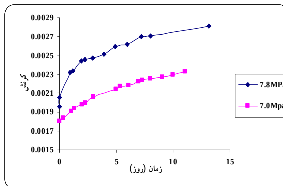
شکل (2) نمودار خزش نمونه‌های ماسه سنگ (تحت تنش‌های مختلف)
