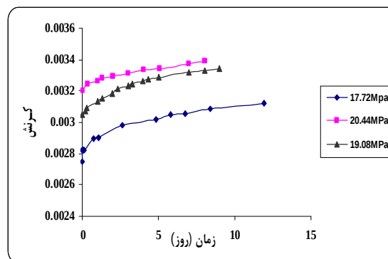
شکل 3 نمودار خزش نمونه‌های گل سنگ (تحت تنش‌های مختلف)
