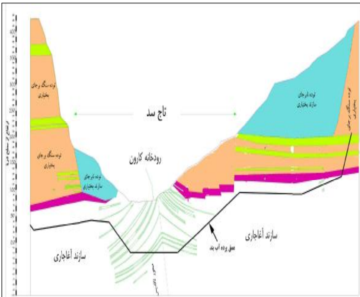
شکل (۱) مقطع زمین‌شناسی ساختگاه سد در جهت محوری سد [۳]
