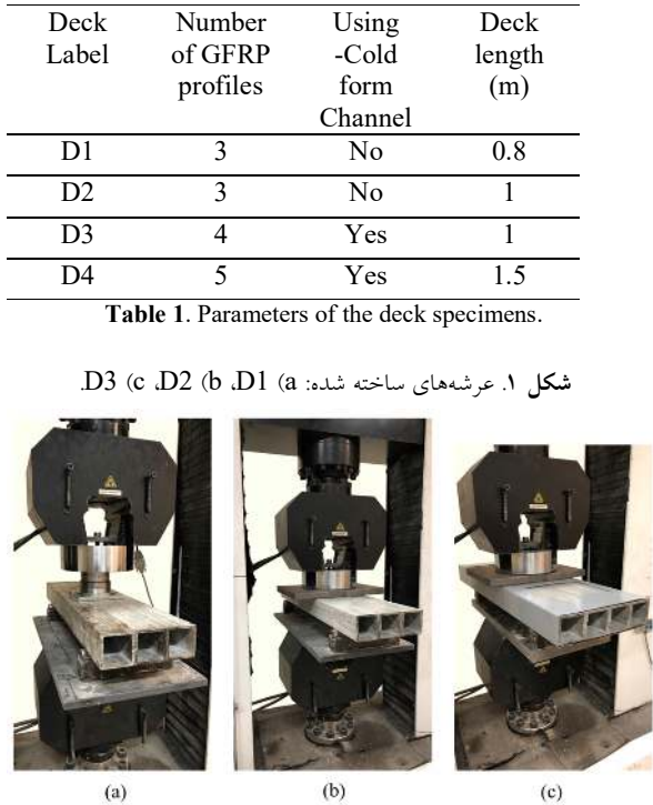
Fig. 1. Deck specimens: a) D1, b) D2, c) D3.
