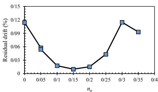
شکل ۱۱. اثر افزایش نسبت نیروی پیش تنیدگی بر جابه جایی نسبی
