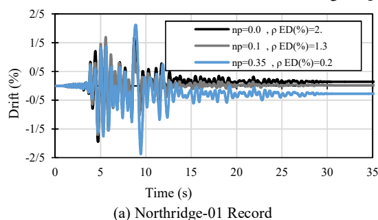
شکل ۱۰. مقایسه تاریخچه جابه جایی نسبی برای نسبت های مختلف پیش تنیدگی
