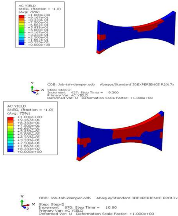
شکل ۲۶. سازوکار خرابی میراگر در زمان‌های مختلف از تحلیل
