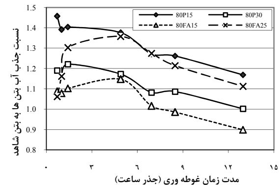
شکل (۹) نسبت جذب آب بتن‌های ۵۰ و ۸۰ حاوی پوزولان طبیعی و خاکستر بادی به بتن شاهد
