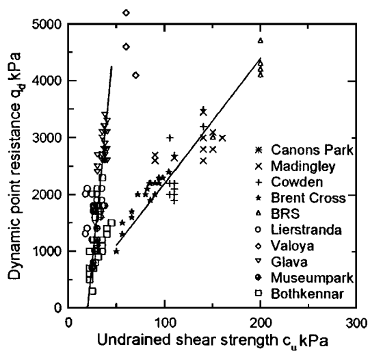
شکل (۷) تغییرات \frac{q_d}{S_v} بر حسب C_u در تحقیق بوچر و همکاران [۳]
