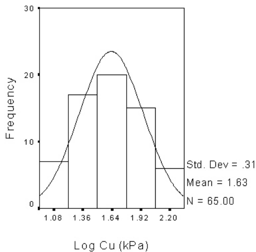
شکل (۸) نمودار تابع توزیع فراوانی C_u
