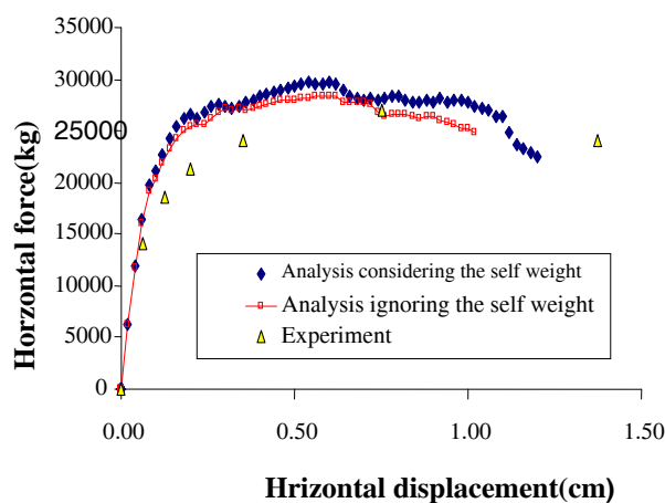
شکل ۱۴ منحنی نیرو - جابجایی دیوار W1
