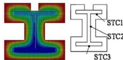
الف) موقعیت ترموکوپل‌ها و کانتور دمای مقطع نمونه C1-S
