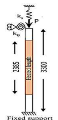
الف) هندسه کلی ستون
