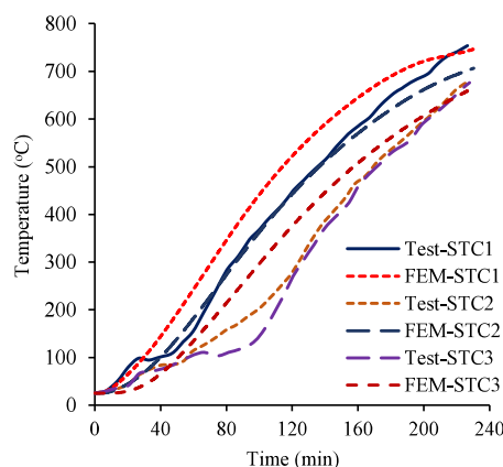
ب) نمودار دما بر حسب زمان نمونه C1-S
