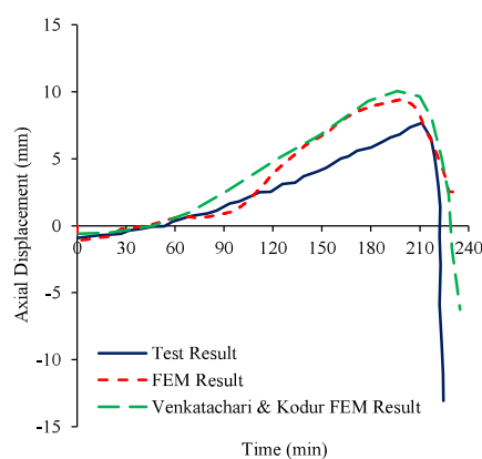
پ) نمودار جابه‌جایی محوری بر حسب زمان نمونه C1-S
