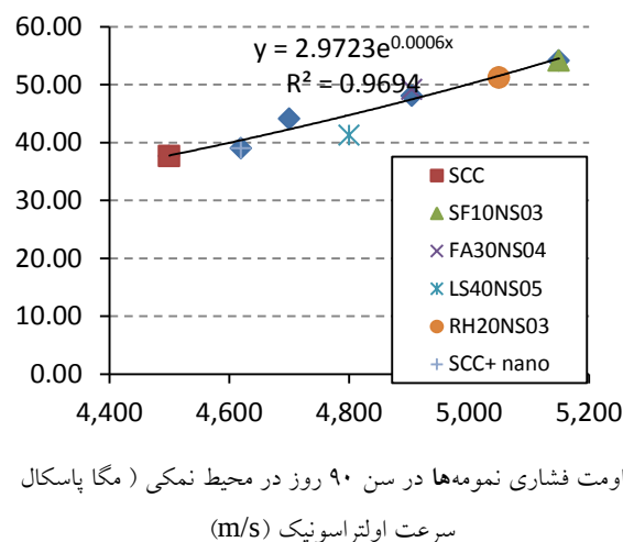
شکل ۷. نمودار مقاومت فشاری نمونه‌ها در برابر سرعت امواج مافوق صوت در محیط کلریدی در سن ۹۰ روز
