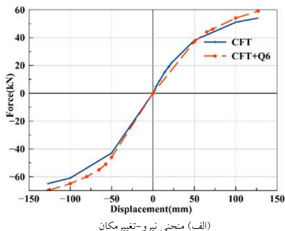
شکل ۱۰. تاثیر شبکه‌های آرماتور افقی در رفتار قاب
