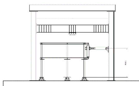
Fig. 2. Test Setup
