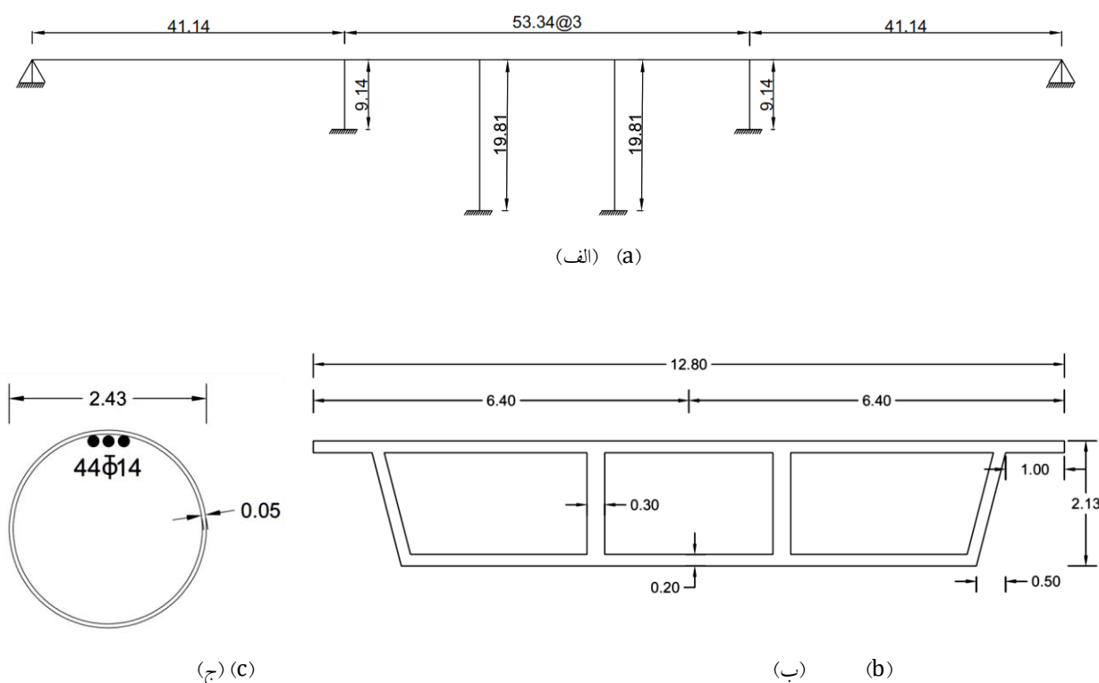
شکل ۱. مشخصات پل TY0H-1 (الف) پروفیل طولی، (ب) مقطع عرضی عرشه و (ج) مقطع پایه پل (ابعاد به متر)
