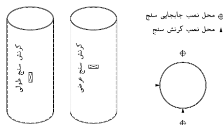
شکل ۵. محل نصب کرنش سنج و جابه‌جایی سنج روی نمونه- نمودار بار به کرنش طولی و عرضی
