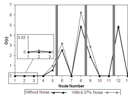
شکل (۱۱) بررسی تاثیر نوفه در سناریوی (۶).
