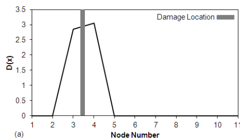
شکل (۳) نتایج حاصل از تشخیص آسیب در سناریوی (۱): (ا): روش پیشنهادی، (ب): روش مبتنی بر انحنای جابه‌جایی استاتیکی [۱۸].
