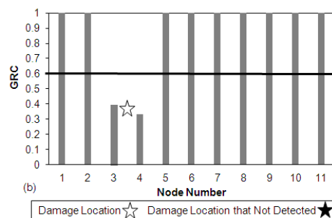
شکل (۳) نتایج حاصل از تشخیص آسیب در سناریوی (۱): (ا): روش پیشنهادی، (ب): روش مبتنی بر انحنای جابه‌جایی استاتیکی [۱۸].
