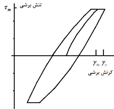
شکل (۱) سیکل تنش - کرنش برشی در مدل موهر کولمب با میرایی هسیتریس
