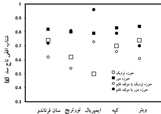
شکل (۱۵) شتاب افقی تاج سد
