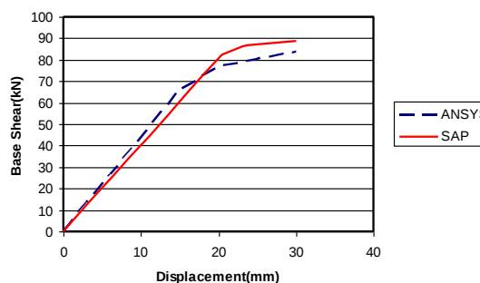
شکل (۱۰): مقایسه پوش و منحنی ظرفیت یک طبقه MS-30%
