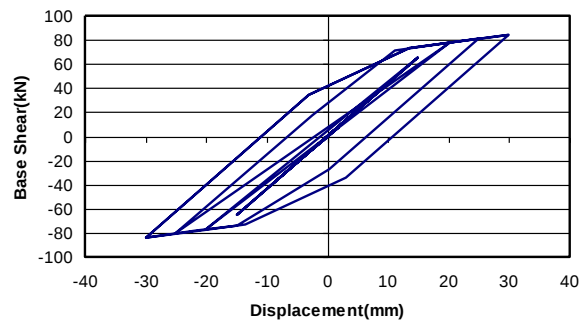
شکل (۶): منحنی چرخه های نمونه یک طبقه MS-30%
