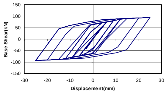
شکل (۵): منحنی چرخه های نمونه یک طبقه LYS-30%
