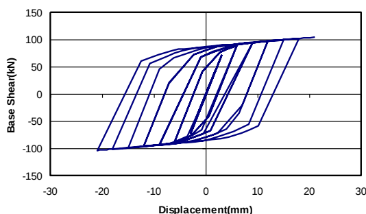
شکل (۳): منحنی چرخه ای نمونه یک طبقه LYS-20%
