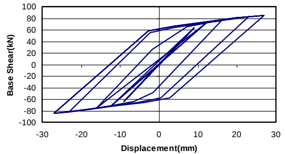
شکل (۴): منحنی چرخه های نمونه یک طبقه MS-20%
