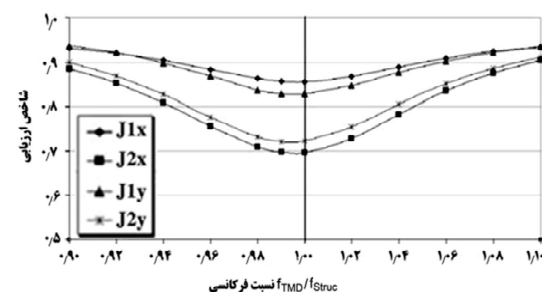
(الف) شاخص‌های ارزیابی پاسخ تغییر مکان
