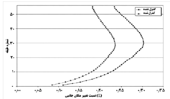
شکل (۸) نسبت تغییر مکان جانبی طبقات در حالت‌های کنترل‌شده و کنترل‌نشده؛ شتاب‌نگاشت بم
