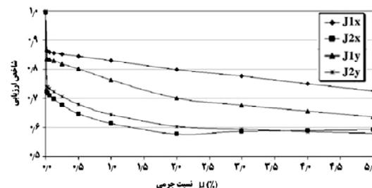
(الف) شاخص‌های ارزیابی پاسخ تغییر مکان
