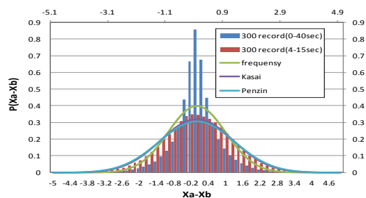
شکل (۱۹): توزیع احتمالاتی تغییر مکان نسبی بین سیستم با شکل پذیری ۴/۵ و ۱/۵
