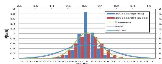
شکل (۱۷): توزیع احتمالاتی تغییر مکان نسبی بین سیستم با شکل پذیری ۲/۵ و ۱/۵
