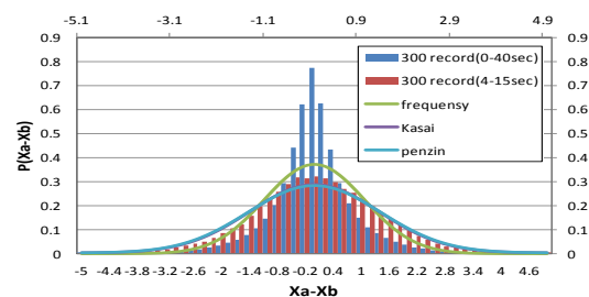
شکل (۲۱): توزیع احتمالاتی تغییر مکان نسبی بین سیستم با شکل پذیری ۲/۵ و ۱/۵
