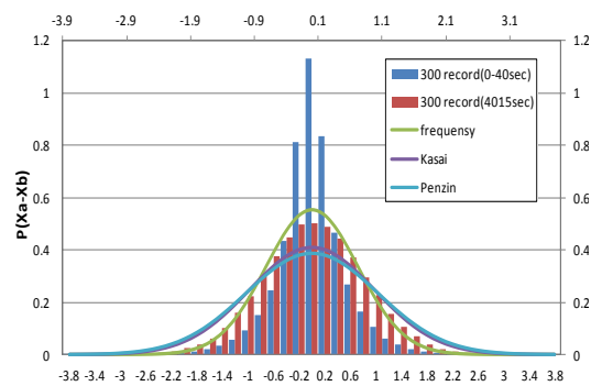
شکل (۱۸): توزیع احتمالاتی تغییر مکان نسبی بین سیستم با شکل پذیری ۳/۵ و ۱/۵
