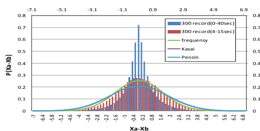
شکل (۲۰): توزیع احتمالاتی تغییر مکان نسبی بین سیستم با شکل پذیری ۵/۵ و ۱/۵
