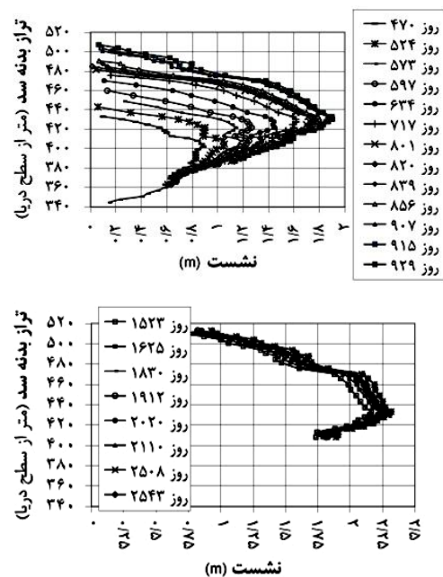
شکل (۱۱) تغییرات نشست نسبت به ارتفاع در هسته‌ی سد در تاریخ‌های مختلف
