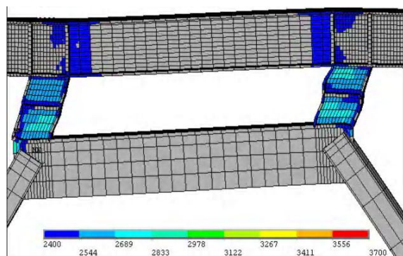
شکل (۹) کانتور تنش فون‌مایسز در دوره آخر بارگذاری برای نمونه SPS1
