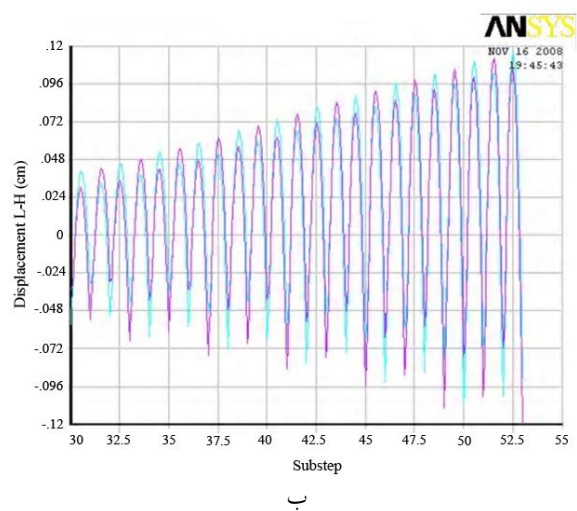
شکل (۱۱) نمودار تغییر مکان دو انتهای پیوند افقی نسبت به سیکل بارگذاری برای نمونه (الف) SPS2 (ب) SPS3
