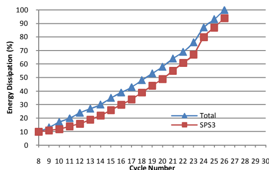
شکل (۱۷) مقایسه سهم پانل برشی نسبت به قاب در استهلاک انرژی
