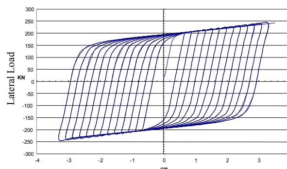
شکل (۷) منحنی هیستریزس برش پایه تغییر مکان نمونه SPS3
