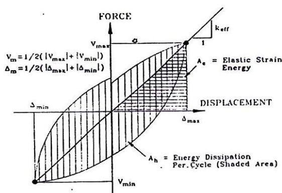
شکل (۱۶) میرایی هیستریزس معادل [۱۳]
