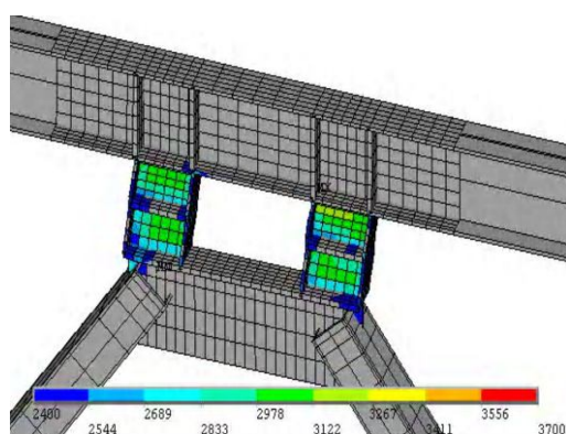
شکل (۱۰) کانتور تنش فون‌مایسز در دوره آخر بارگذاری برای نمونه SPS3
