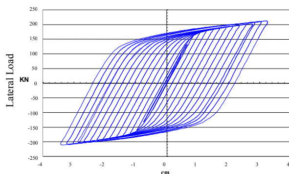
شکل (۶) منحنی هیستریزس برش پایه تغییر مکان نمونه SPS2
