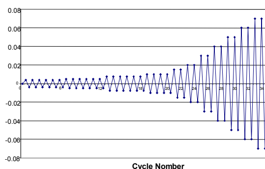
شکل (۳) نمودار بارگذاری چرخه‌ای طبق روند AISC ۲۰۰۵ [۱۲]
