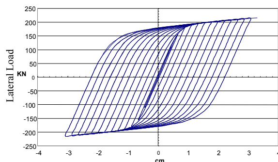
شکل (۵) منحنی هیستریزس برش پایه تغییر مکان نمونه SPS1
