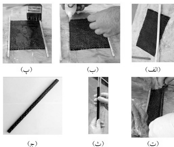
شکل (۲) فرایند ساخت میل‌های BMCF
