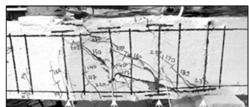
(ج): نمونه VBA-W
