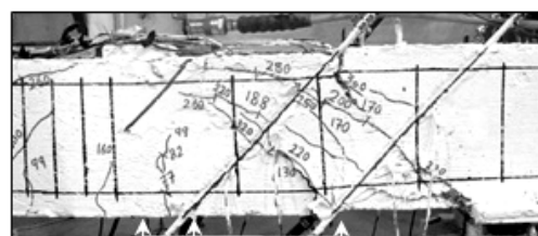
(پ): نمونه IB
