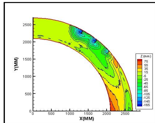
شکل (۴) نمونه‌ای از توپوگرافی بستر برداشت شده توسط دستگاه لیزری برداشت پروفیل بستر در قوس ۹۰ درجه با آبشکن T شکل
