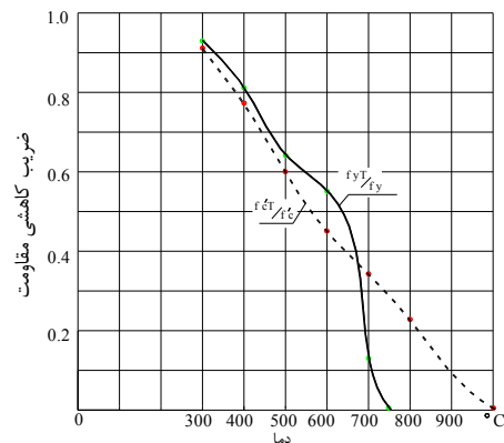
شکل (۳) تأثیر دما بر میزان مقاومت مشخصه بتن و تنش تسلیم فولاد [۱۶]
