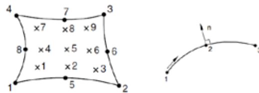
شکل ۴ المان‌های اجزاء محدود (الف) المان خرپای دو بعدی (ب) المان دو بعدی تنش مسطح
