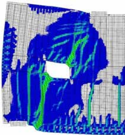
شکل ۲۳ مود شکست برشی در تیر عمیق با آرماتور قائم
