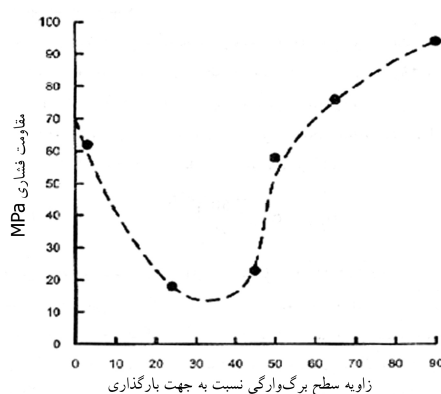
شکل (۸) مقاومت فشاری تک محوری در مقابل زاویه سطح برگرادگی نسبت به جهت برگرادگی.
