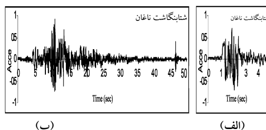
شکل ۶ شتابنگاشت مربوط به (الف) زلزله ناغان (ب) زلزله طبس
