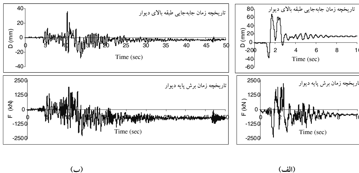
شکل ۷ نمودارهای تاریخچه زمانی دیوار ۵ طبقه با ارتفاع تیر ۱۰۰ سانتیمتر مربوط به: (الف) زلزله ناغان (ب) زلزله طبس
