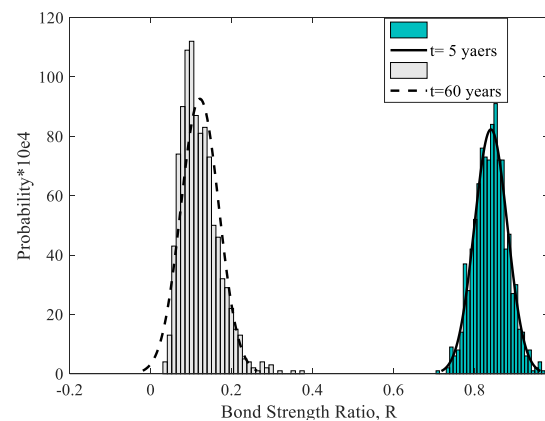
شکل ۱۵. هیستوگرام و تابع چگالی احتمال برای میلگرد به قطر ۱۲ تحت اثر چگالی جریان خوردگی ۳ میکروآمپر با ضریب تغییرات ۰/۳
