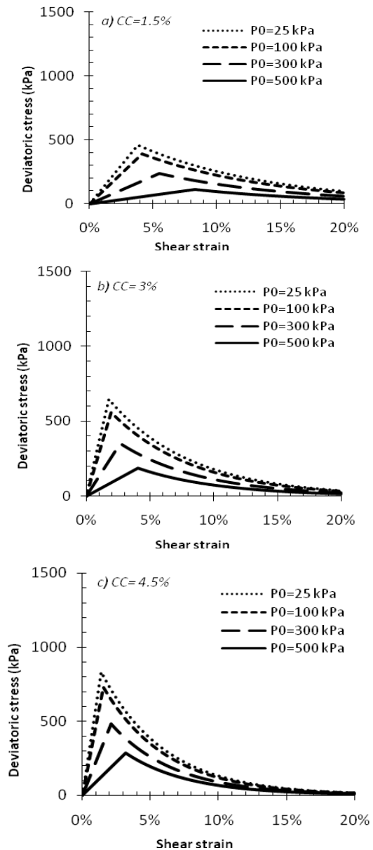
شکل (۳) منحنی تنش-کرنش باندهای سیمانی با فشارهای همه جانبه مختلف و درصد‌های مختلف سیمان در شرایط زهکشی شده CC=۱/۵ (a) CC=۳/۳ (b) CC=۴/۵ (c)
