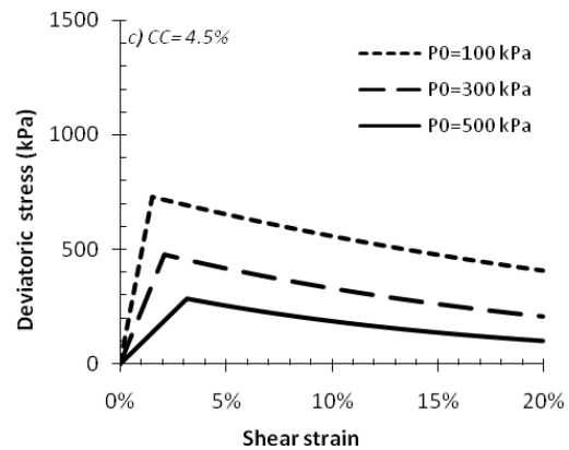
شکل (۸) منحنی تنش-کرنش باندهای سیمانی با فشارهای همه جانبه مختلف و درصدهای مختلف سیمان در شرایط زهکشی نشده CC=۱/۵ (a) CC=۳/۳ (b) CC=۴/۵ (c)
