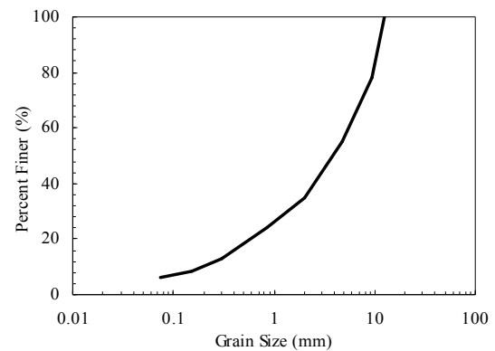
شکل (۱) منحنی دانه‌بندی خاک ماسه‌ای [۲۵]
