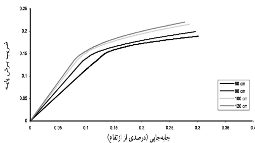
شکل ۵ نمودار بار - تغییر مکان بالای دیوارهای ۵ طبقه با ارتفاع های مختلف تیر تحت بار جانبی افزایشی
