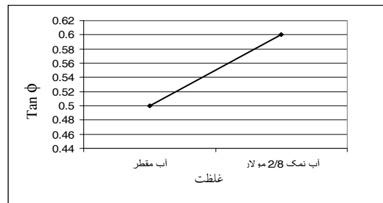
شکل ۱۱ نمودار تغییرات تانژانت زاویه اصطکاک داخلی در مقابل تغییرات غلظت سیال حفره‌ای
