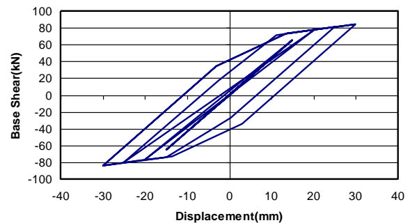
شکل (۸): مقایسه پوش و منحنی ظرفیت یک طبقه MS-30%
