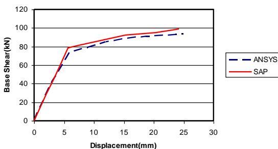
شکل (۵): مقایسه پوش و منحنی ظرفیت یک طبقه LYS-30%
