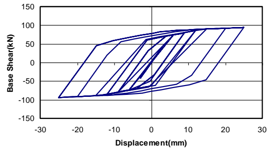
شکل (۷): مقایسه پوش و منحنی ظرفیت یک طبقه LYS-30%
