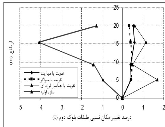
شکل (۱۴) تغییر مکان نسبی طبقات بلوک دوم شده در تحلیل دینامیکی غیرخطی تحت زلزله بم
