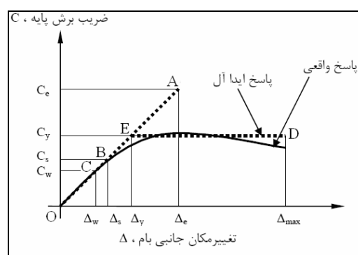
شکل ۱ پاسخ کلی سازه‌ها در برابر زلزله‌های شدید
