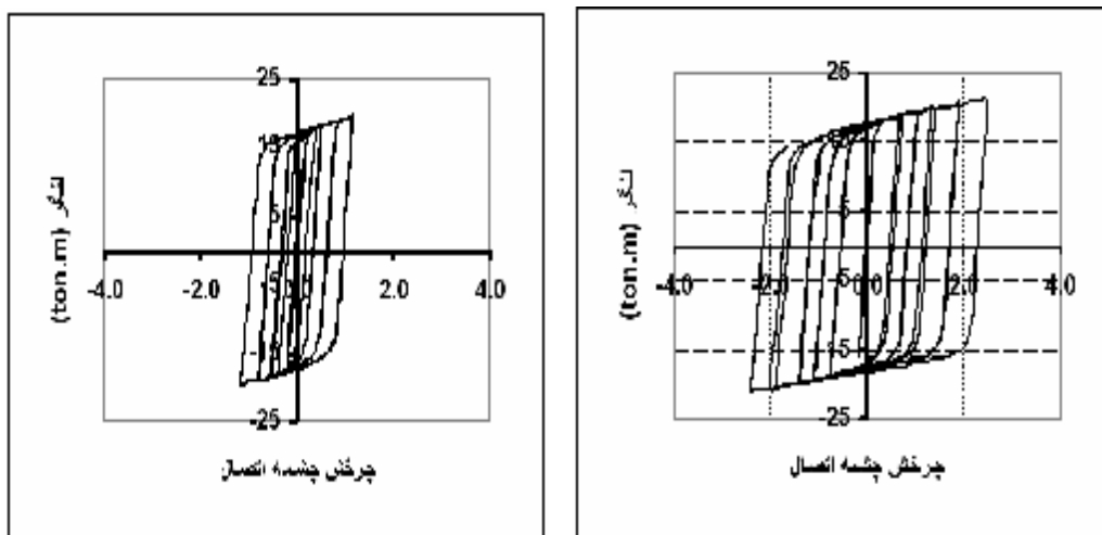
شکل (9) منحنی لنگر - چرخش برای چشمه اتصال نمونه‌های تحلیل شده؛ الف ( نمونه SMF، ب ) نمونه RBS
