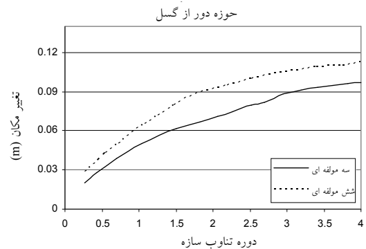
شکل (۱۱) تغییرات جابه‌جایی نسبت به تناوب سازه نامتقارن برای زلزله‌های حوزه نزدیک و دور e_s / \beta = 40\%
