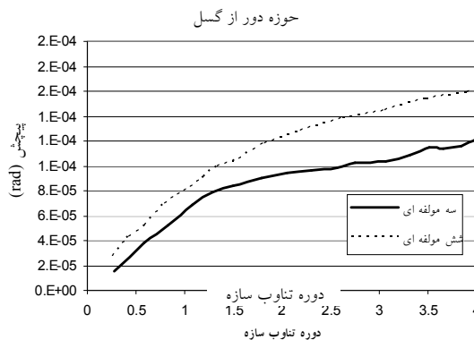
شکل (۱۲) تغییرات پیچش نسبت به تناوب سازه نامتقارن برای زلزله‌های حوزه نزدیک و دور e_s / \beta = 40\%
