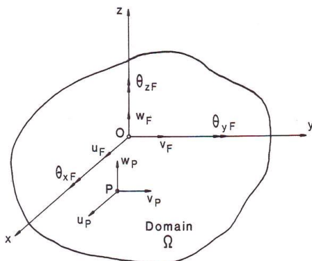
شکل (۳) نمایش میدان آزاد حرکت زمین [۳]
