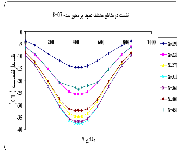
شکل 10 تغییرات نشست در مقاطع مختلف عمود بر محور سد با تغییر مقدار K=0/7
