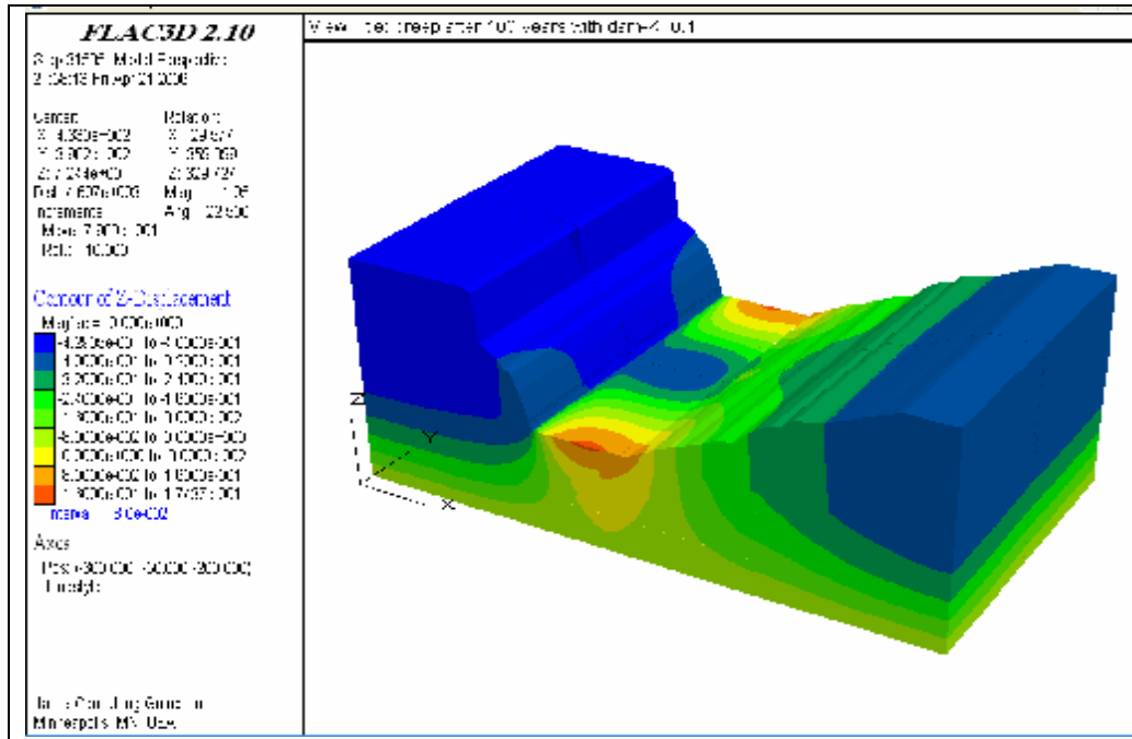
شکل 11 خطوط تراز جابجایی‌های عمودی پس از خزش 100 ساله همراه با سد بر حسب متر برای K=0/55
