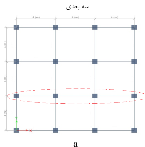
شکل ۴. هندسه سازه ۹ طبقه a-پلان b-نمای قاب دوبعدی c-ساختمان
