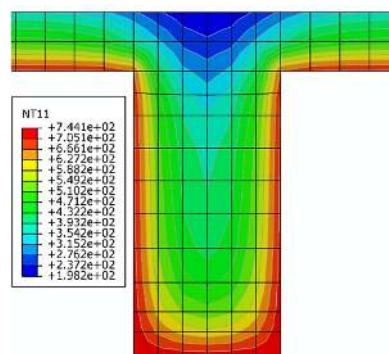
(ب) تیر با مقطع 350×150
