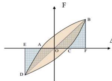
شکل ۲۰. نمونه حلقه هیستریزس متعارف [14].
