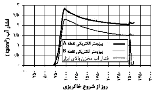
شکل (۴) تغییرات فشار آب حفره‌ای نسبت به زمان در نقاط A و B
