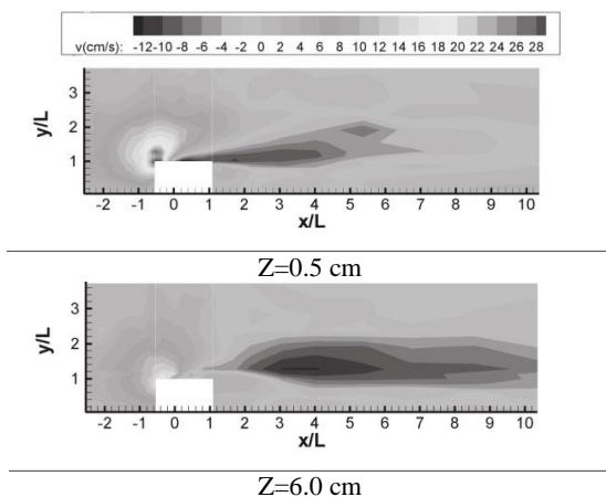
شکل (۵) توزیع مؤلفه عرضی سرعت در ترازهای مختلف قائم
