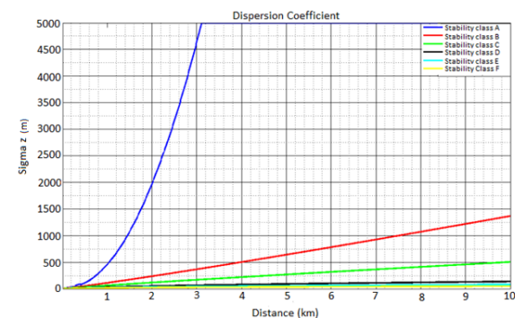
شکل ۳: ضریب پراکندگی گوس در جهت عمودی برای کلاس‌های پایداری مختلف
