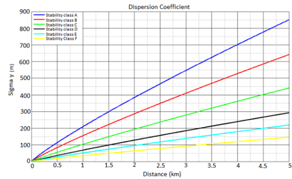
شکل ۲: ضریب پراکندگی گوس در جهت مایل برای کلاس‌های پایداری مختلف.
