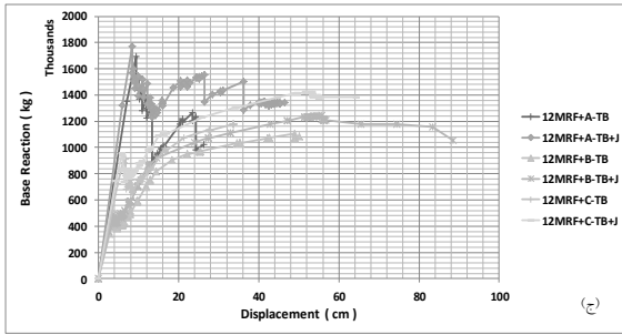
شکل (۱۲) منحنی‌های نیرو-تغییر مکان مدل‌های ۱۲ طبقه قاب خمشی با مهاربند کماتش تاب (الف) و معمولی (ج) در سه تیب A ، B و C ، مدل‌های قاب خمشی تنها، قاب خمشی با مهاربند معمولی و کماتش تاب تیب B (ب)، به همراه حالت افزودن زره پوش بتنی به آنها
