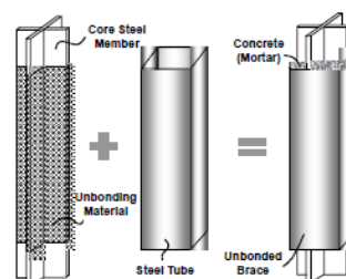
شکل (۱) نمایی شماتیک از مهاربند کمانش تاب [۱]
